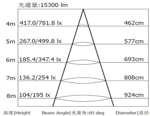
照度图 Illuminance map
