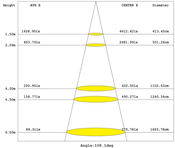
照度图 Illuminance map
