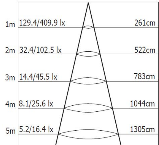
照度图 Illuminance map
